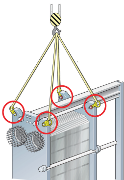
Bild 7: Lyftanordning för AQ18 och AQ14L. Säkringsutrustning krävs inte.
