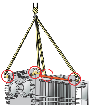
Bild 8: Lyftanordning för AQ20. Säkringsutrustning krävs.
