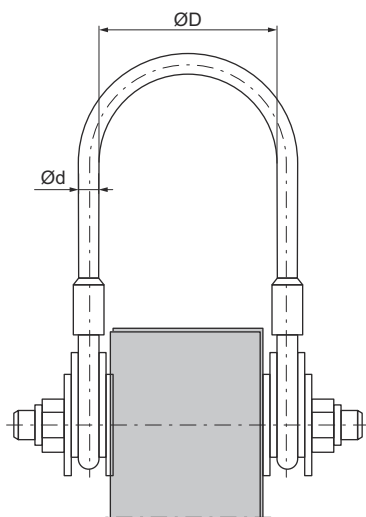
Bild 5: Lyftvajer monterad med en ramplatta.
