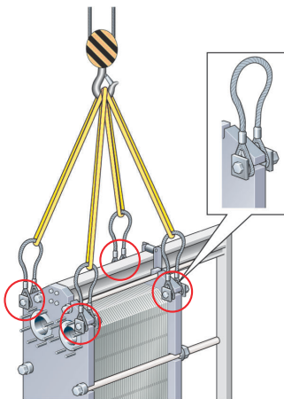
Bild 6: Lyftanordning för AQ14 och AQ14S. Säkringsutrustning krävs.
